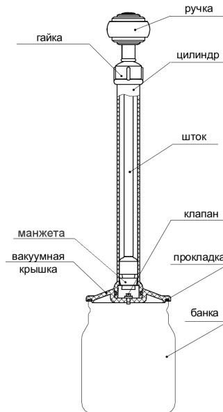
Рис.1. Схема работы вакуумного насоса
